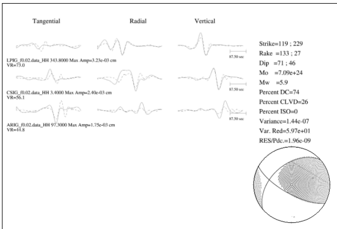
Figura 3. Mecanismo focal del sismo del 27 de mayo de 2025, magnitud 5.9.
