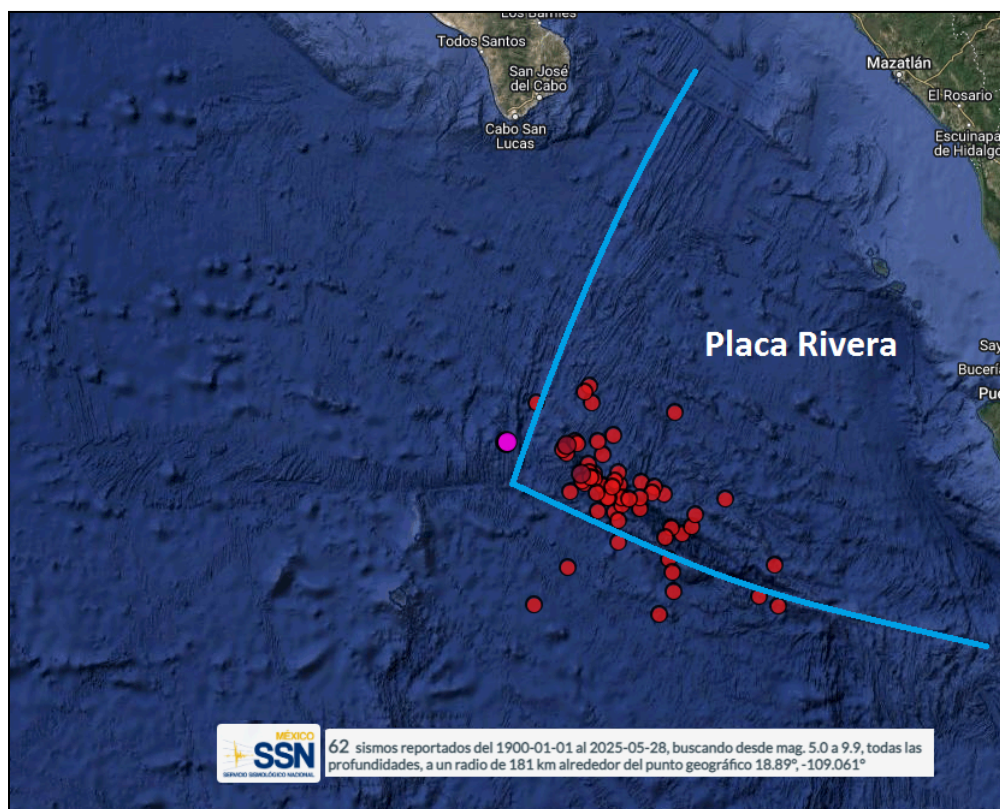
Figura 4. Sismicidad histórica localizada en la zona de placa Rivera.
