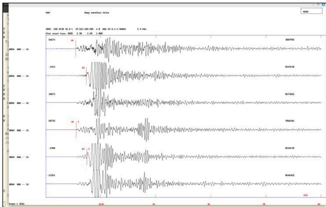
Figura 2. Registros sísmicos en las estaciones de banda ancha del Servicio Sismológico Nacional en la Isla Socorro.
