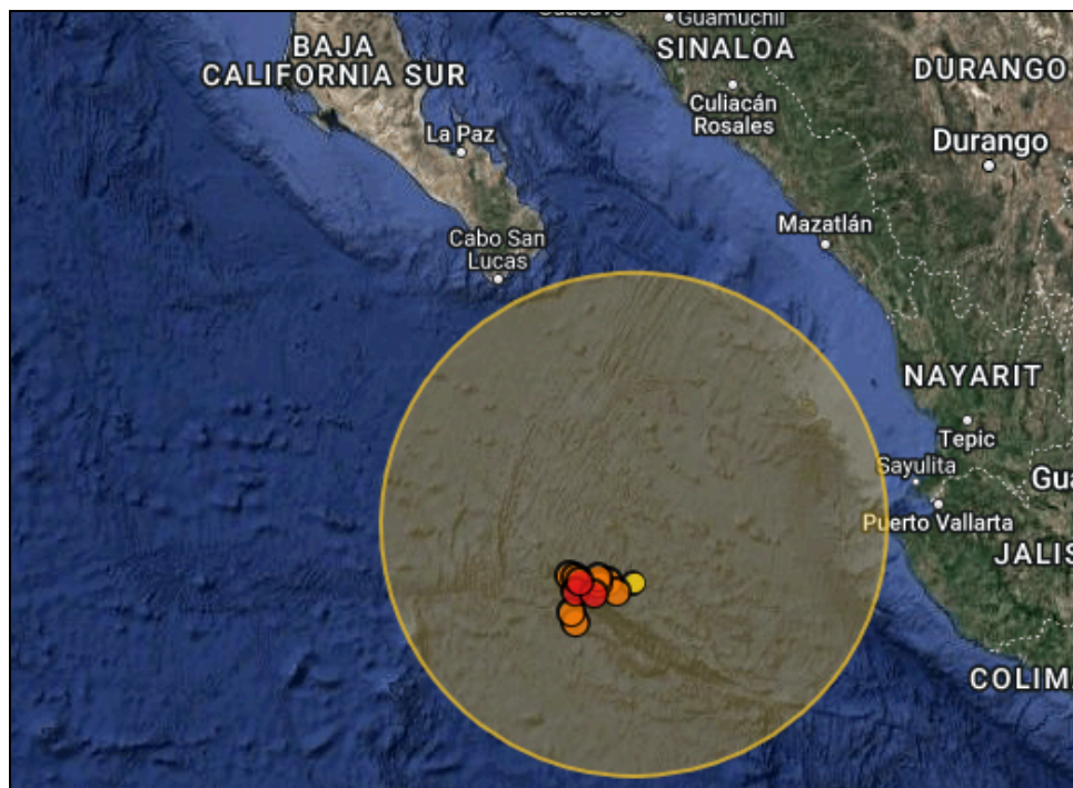
Figura 1. Epicentros de los sismos que conforman la secuencia del 27 y 28 de mayo de 2025.
