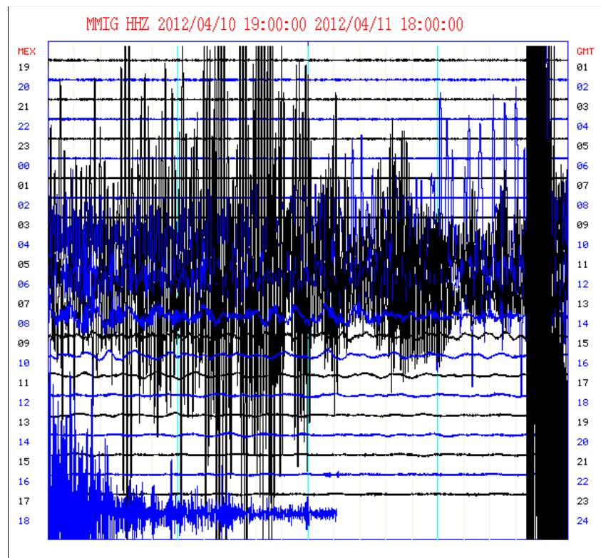
Figura 2. Sismograma de la estación de Banda Ancha de Maruata, Michoacán (MMIG). (Este registro es de un telesismo real y se muestra únicamente como ejemplo)
