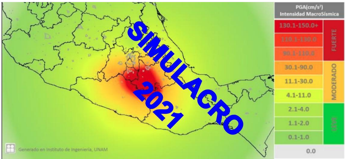
Figura 4. Mapa de intensidades del temblor ficticio del simulacro del día 19 de septiembre de 2021. Este mapa fue generado por el Instituto de Ingeniería de la UNAM .
