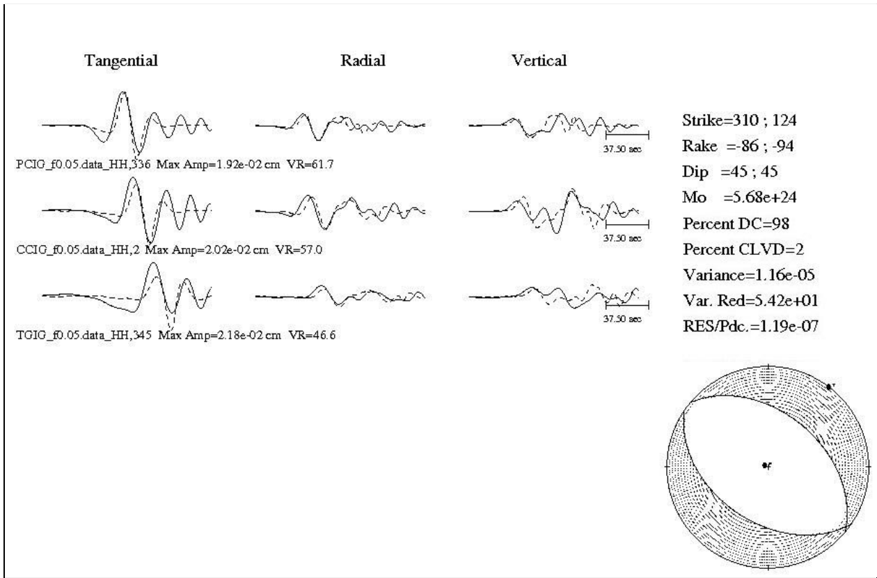
Figura 3. Mecanismo focal del sismo ficticio del simulacro del día 19 de septiembre de 2021. (El mecanismo que se ve en la figura es de un sismo real y se muestra únicamente como ejemplo).
