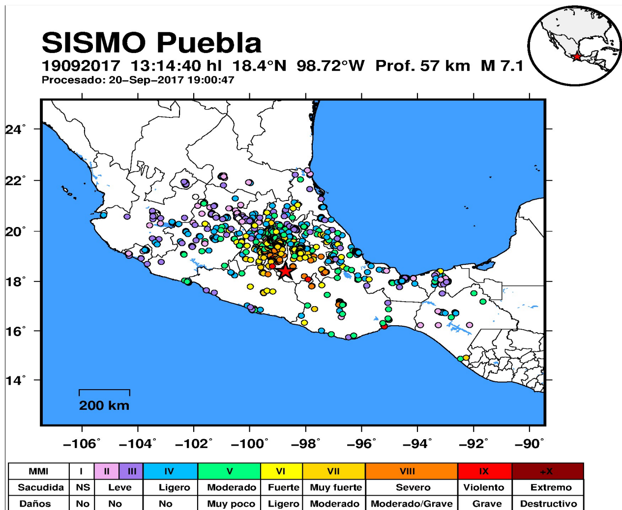
Figura 5. Mapa de intensidades macrosísmicas del sismo ficticio del macrosimulacro 2021. Este mapa se genera con información proporcionada por la comunidad de internet y lo elabora la Universidad Autónoma de Nuevo León, Facultad de Ciencias de la Tierra. (Este mapa se generó para un evento sísmico real y se muestra sólo como ejemplo).
