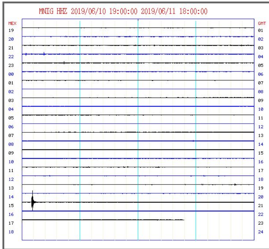
Figura 2. Registro sísmico en la estación de banda ancha del Servicio Sismológico Nacional ubicada en Monterrey, del temblor del día 11 de junio de 2019.
